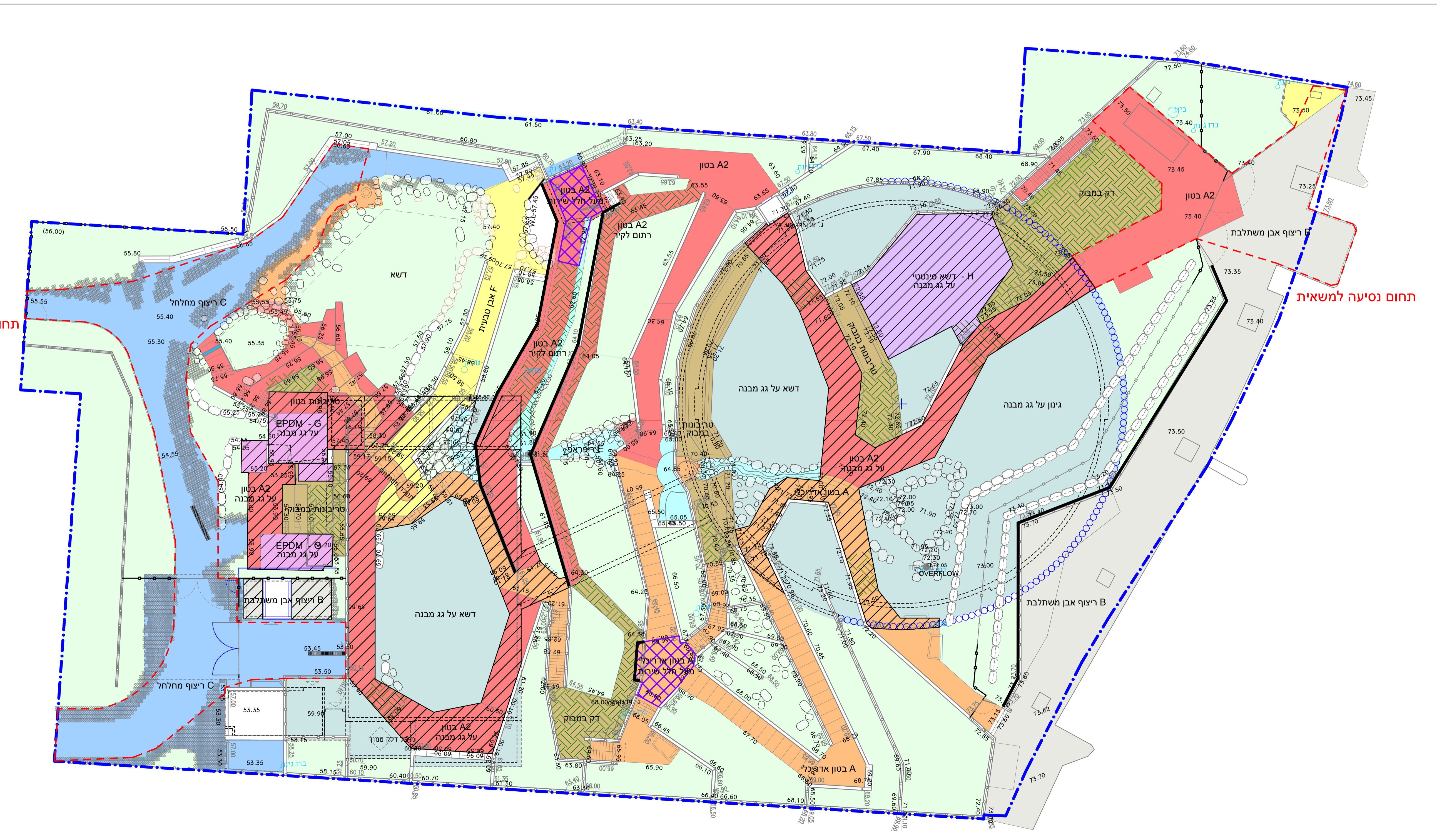
מקרא תכנית מבנה תת-קרקעי 1:200
