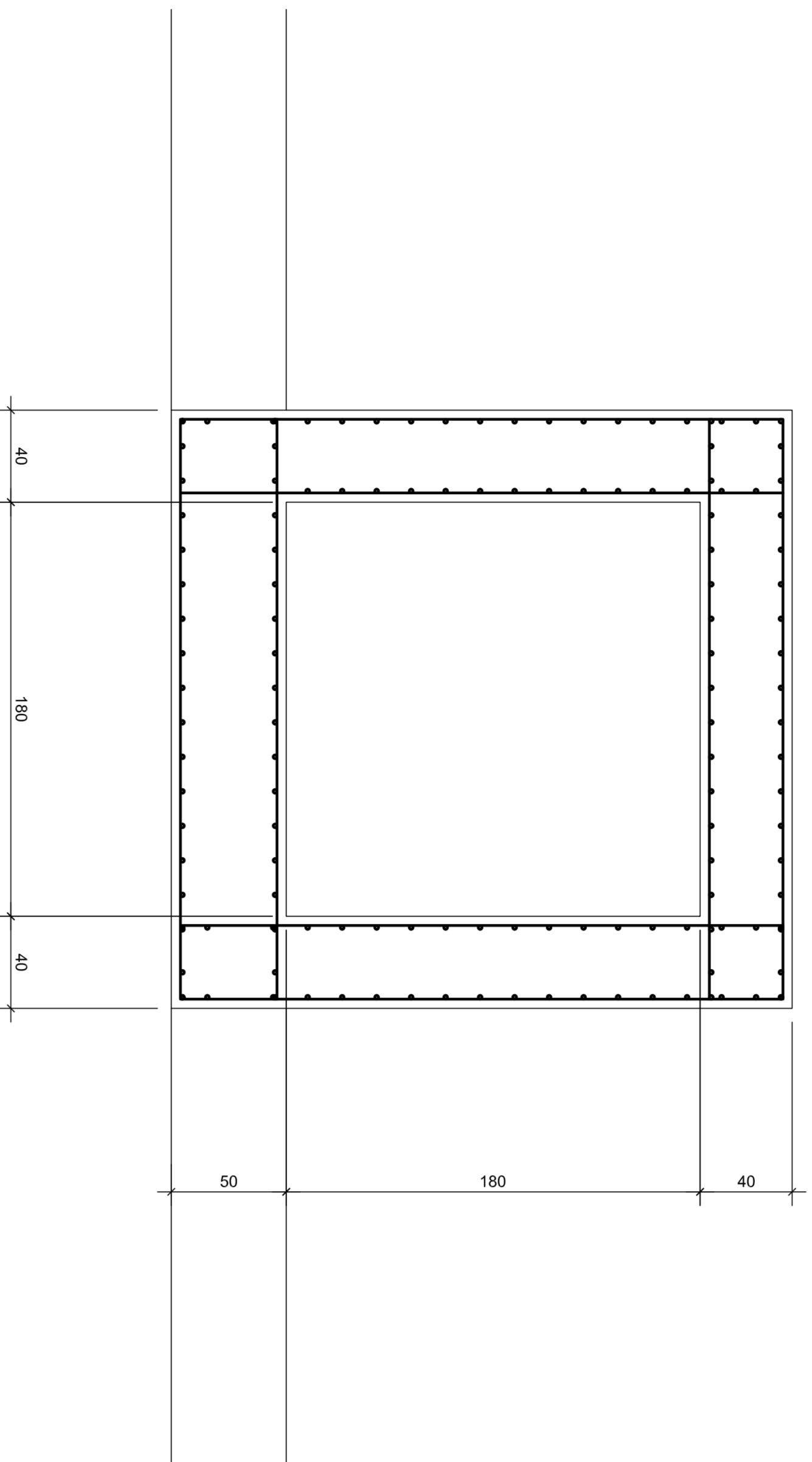
תוכנית השולחן 1:20
